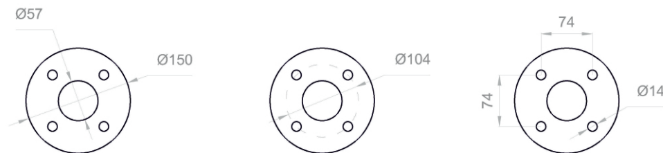
Фланец 150/5
